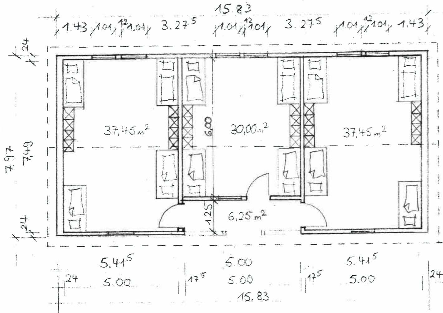
GRUNDRISS
